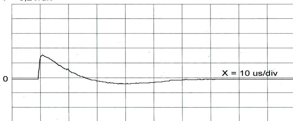
Obr. 10 Oscilogram napět'ové odezvy na výstupu KPO se zkratovaným čtvrtvlnným vedením
